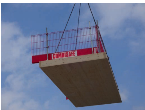
Montage préalable de la protection latérale
