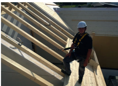
Exemple point B: ABS-Lock DH04 d'après EN795
