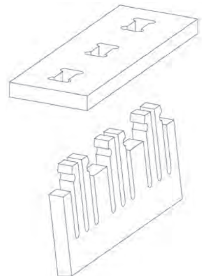
↘ Schéma du principe de joint développé par l'IBOIS
