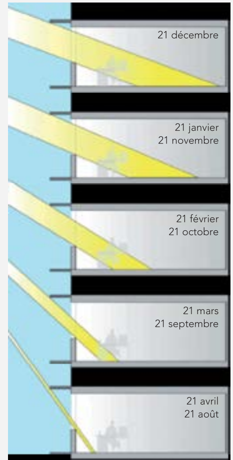
↑ Figure 4 Exemple de façade orientée sud protégée d'un auvent fixe, vis-à-vis du rayonnement solaire selon les saisons (de haut en bas de l'hiver à l'été) – Source ESTIA- cahier pratique du moniteur : fenêtres, dimensionnement et performances.
