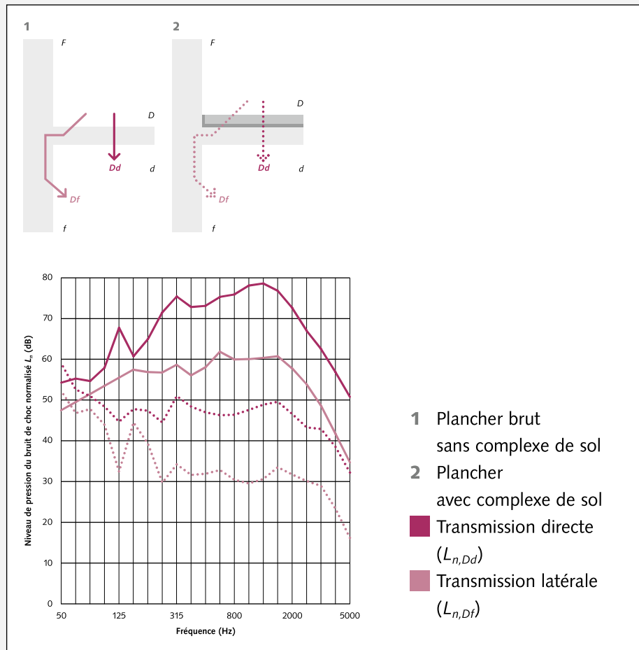
↑ Figure 4 Extrait documentation Lignum Influence d'un complexe de sol sur la transmission directe (voie Dd) et sur les transmissions latérales (voie Df) des bruits de choc entre deux locaux superposés : plancher (plancher à caissons) directement relié aux parois porteuses (ossature bois).
