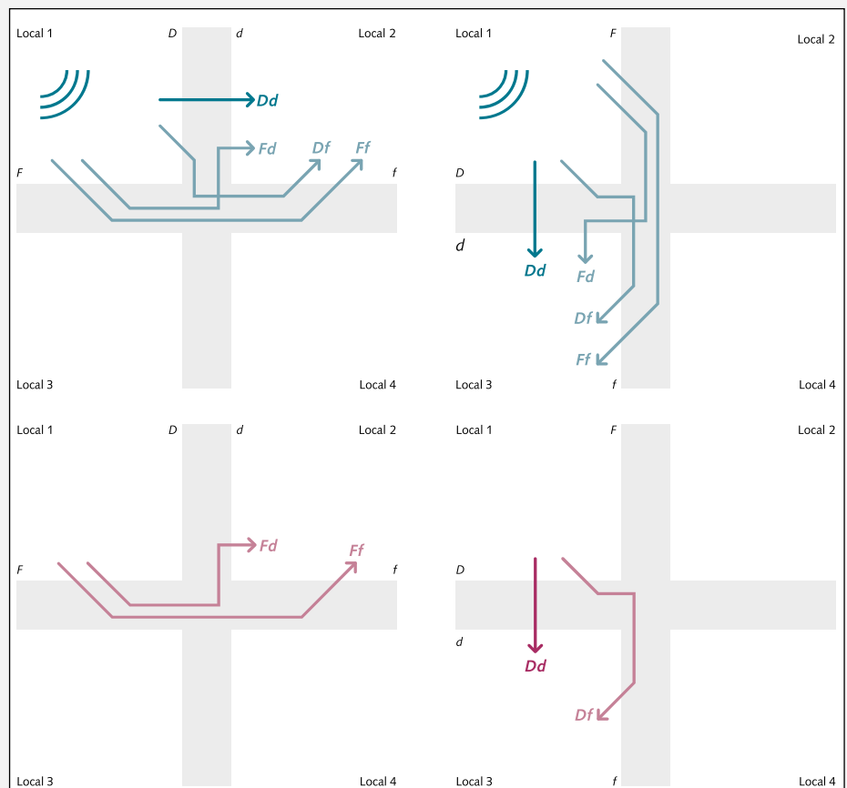
↑ Figure 3 Schéma de principe et de repérage des différentes voies de transmission du son à une jonction en X plancher / paroi. En haut : bruits aériens. En bas : bruit de choc Source : documentation Lignum
