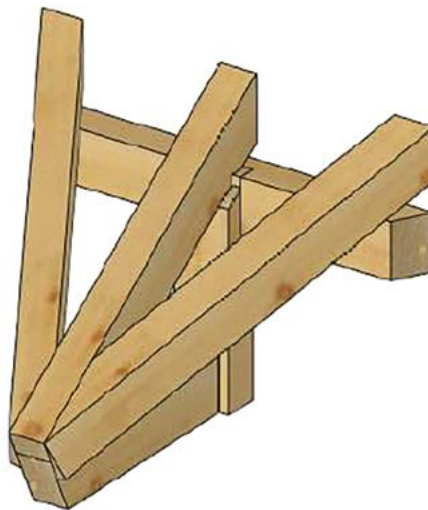
↓ Exemple de maquette réalisée en charpenterie durant les championnats de section
