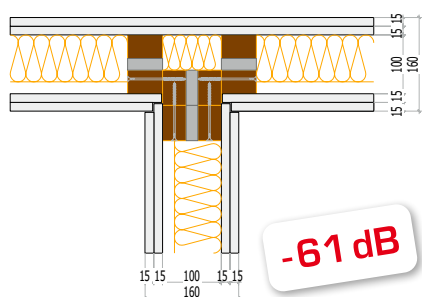
Détail raccord entre 2 séparations
