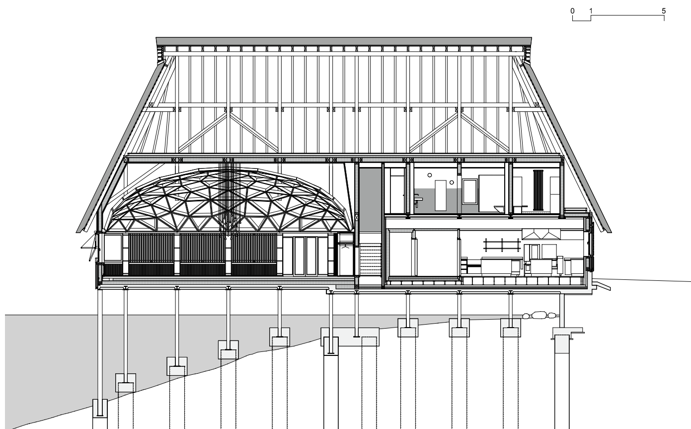
↓ Plan transversal de la Fischerstube
