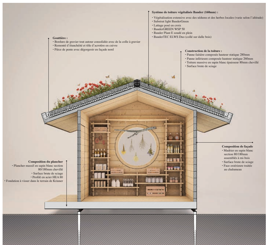
↑ Vision transversale de Maïsatte – holaa Bienne (BE)
