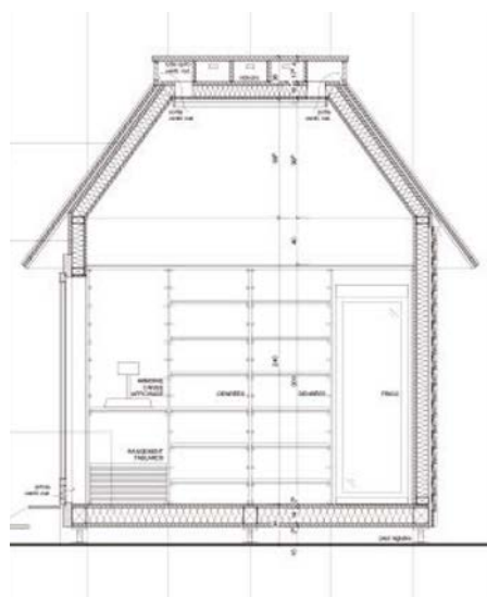
↑ Coupe transversale du projet Les Arches – ERBAT Architectes SA, La Sarraz (VD)
