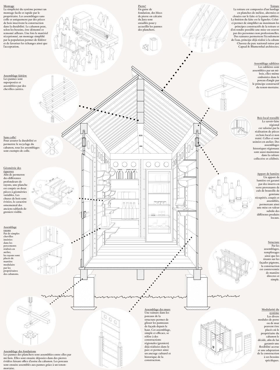
↑ Détails du cabanon Chassrrral – APOLLO Architecture Sàrl, Bienne (BE)
