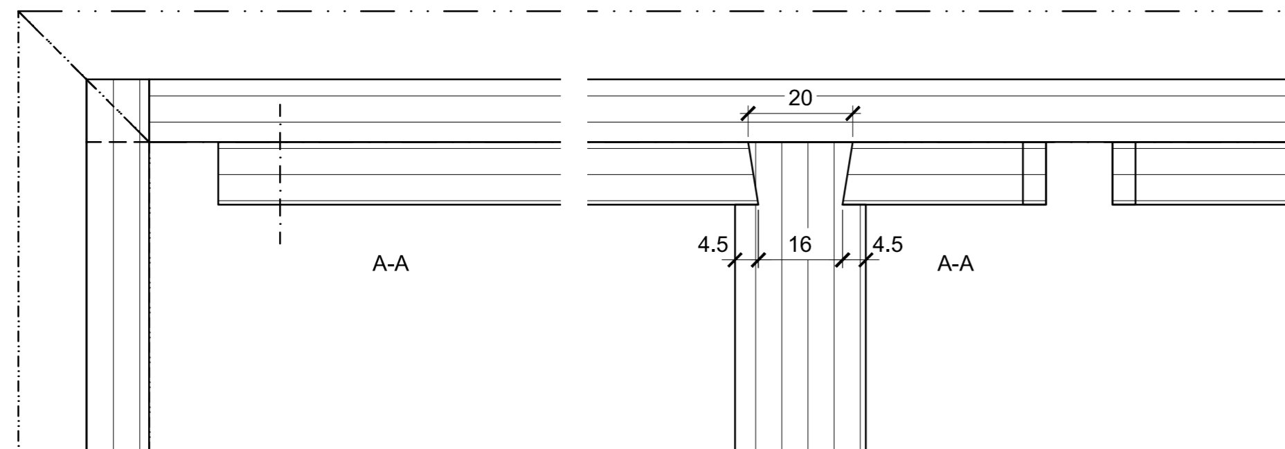
Vue de la traverse du cadre
