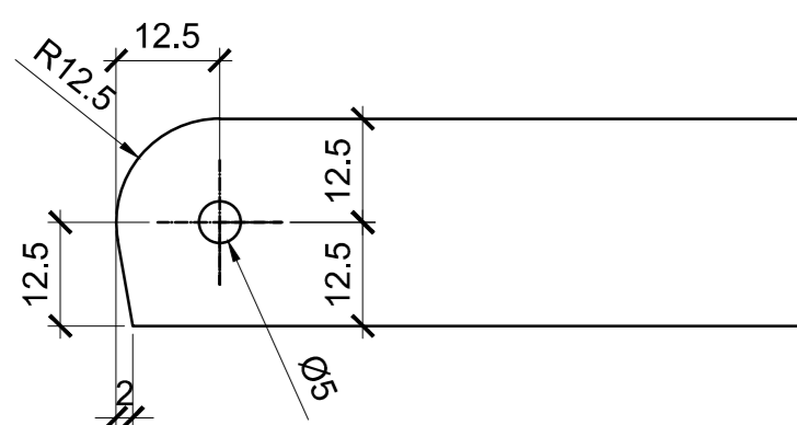
Vue du haut du pied
