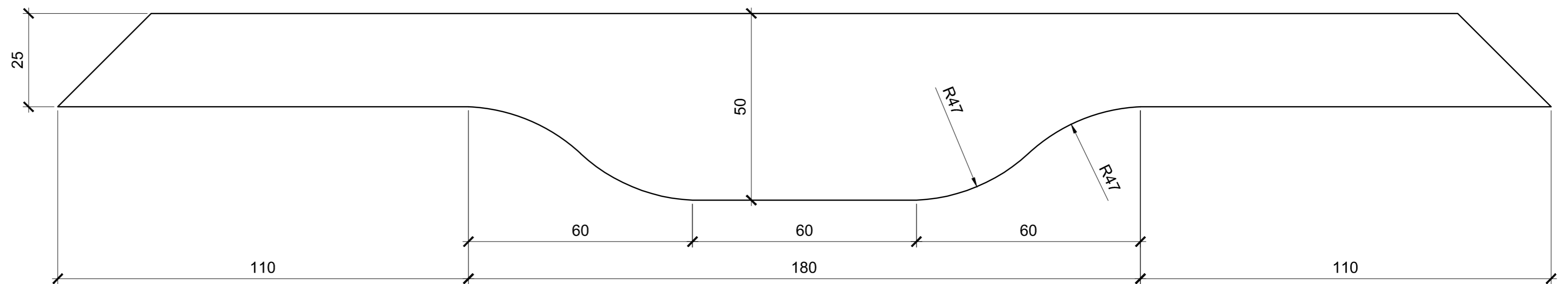
Vue de la traverse du cadre
