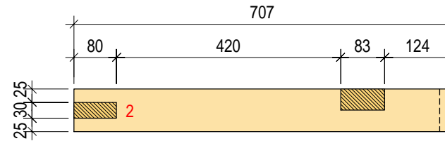
VUE COUPE A -- A
