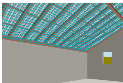
1 Filet de sécurité en tant que protection collective au-dessous de l'ensemble de la surface du toit.
