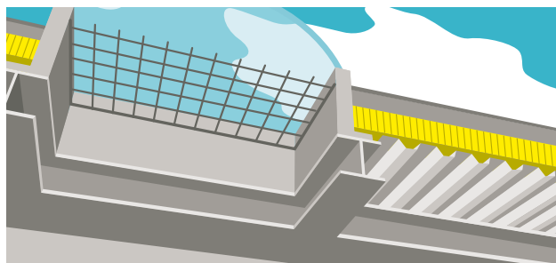
2 Ouverture de toit (puits de lumière) avec grille de protection fixe.
