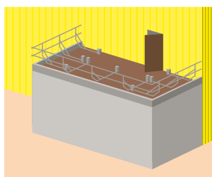
2 Toit plat avec garde-corps temporaire.
