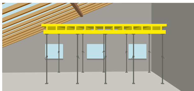
2 Échafaudage de retenue en construction. Il doit encore être prolongé pour protéger toute la zone de chute.
