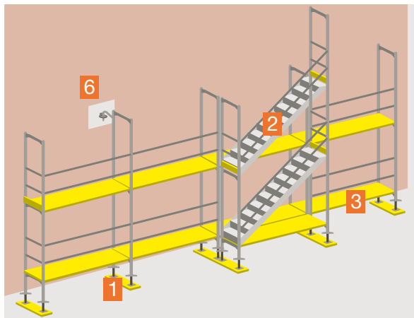
1 Points à contrôler pour les échafaudages
