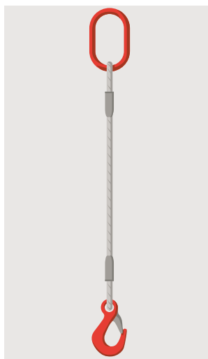
1 Élingue câble à un brin
