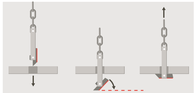
5 Jeu de chaîne à un brin pour plaques d'acier
