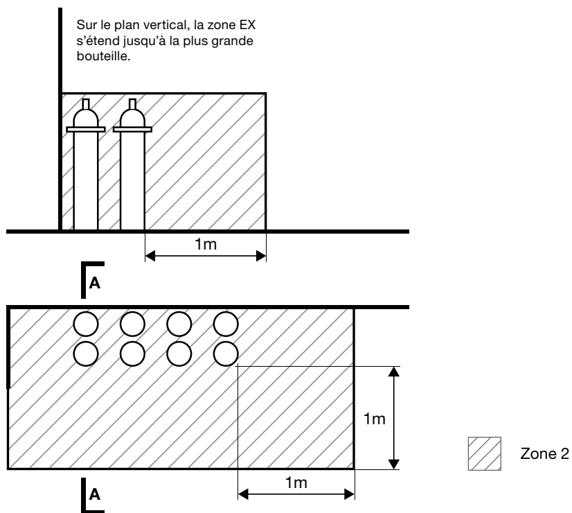
Coupe A-A
